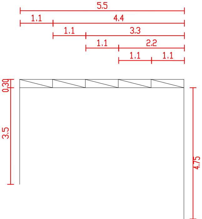
2D: VISTA LATERAL TRELIÇA
